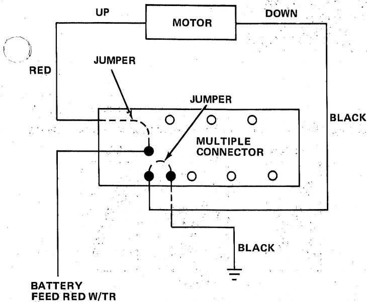
Fig. 3J-8 Motor Switch UP Test
